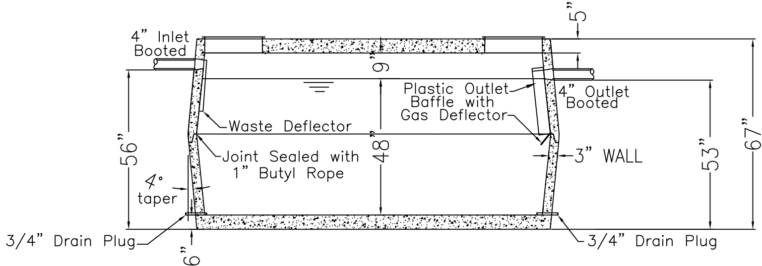
SECTION A-A
